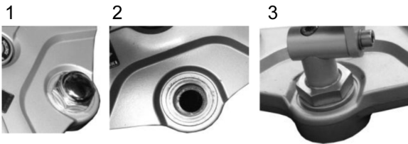
NL : Vervang de kroonplaatmoer door de bijgeleverde kroonplaatmoer. advies: Laat dit door Uw Dealer uitvoeren. GB : Replace the center Bolt with the nieuw delivered center Bolt. advice : Let your Dealer do this. D : Ersetz die Lenkkopfmutter mit die neue Lenkkopfmutter . Rat : Überlegen mit die Dealer.
